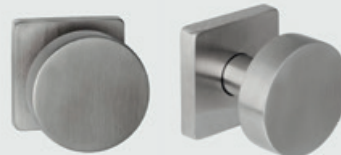
Scheibenknopf auf Q-Rosette Edelstahl matt, Durchmesser 50 mm; Rosettenmaße: 10 x 52 x 52 mm
